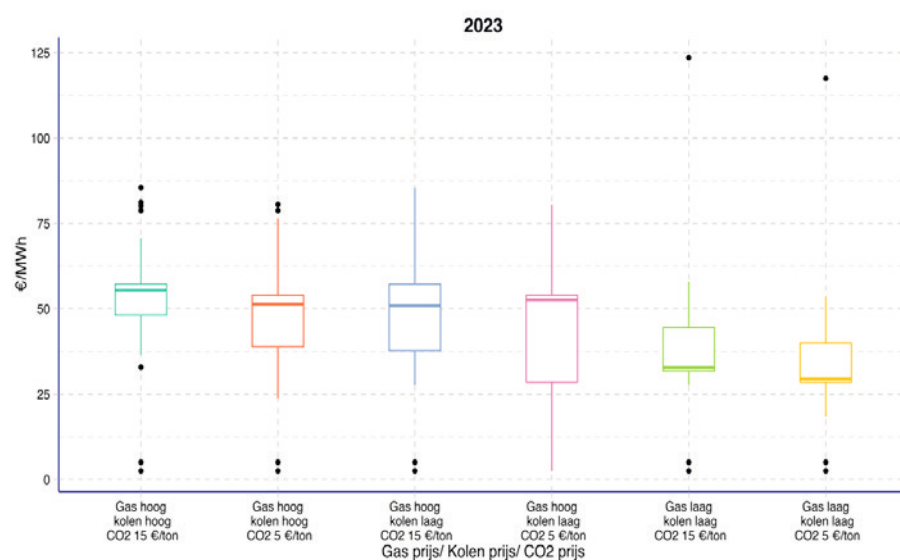
Figuur B1.13. Gemiddelde elektriciteitsprijzen en volatiliteit bij verschillende commodityprijzen (2023).
